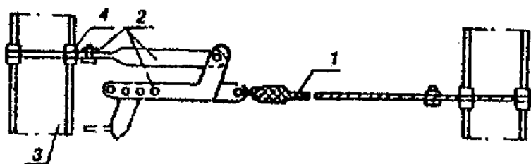
Принципиальная схема установки страховочного каната
