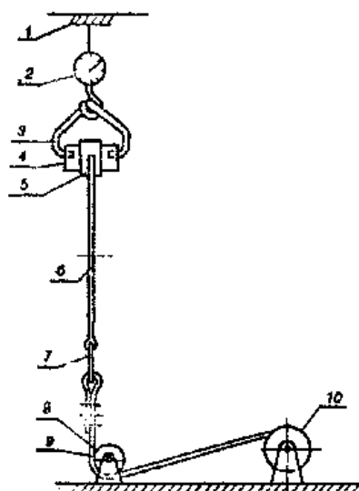
1 — опора; 2 — динамометр; 3 — захват специальный; 4 — ролик цилиндрический; 5 — пояс; 6 — строп; 7 — карабин; 8 — канат тягловый; 9 — блок направляющий; 10 — лебедка
