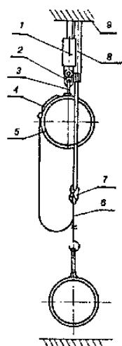
1 — устройство расцепляющее; 2 — серва резачная; 3 — кольцо пояса; 4 — груз; 5 — пояс; 6 — строп; 7 — карабин; 8 — штанга; 9 — опора жесткая
