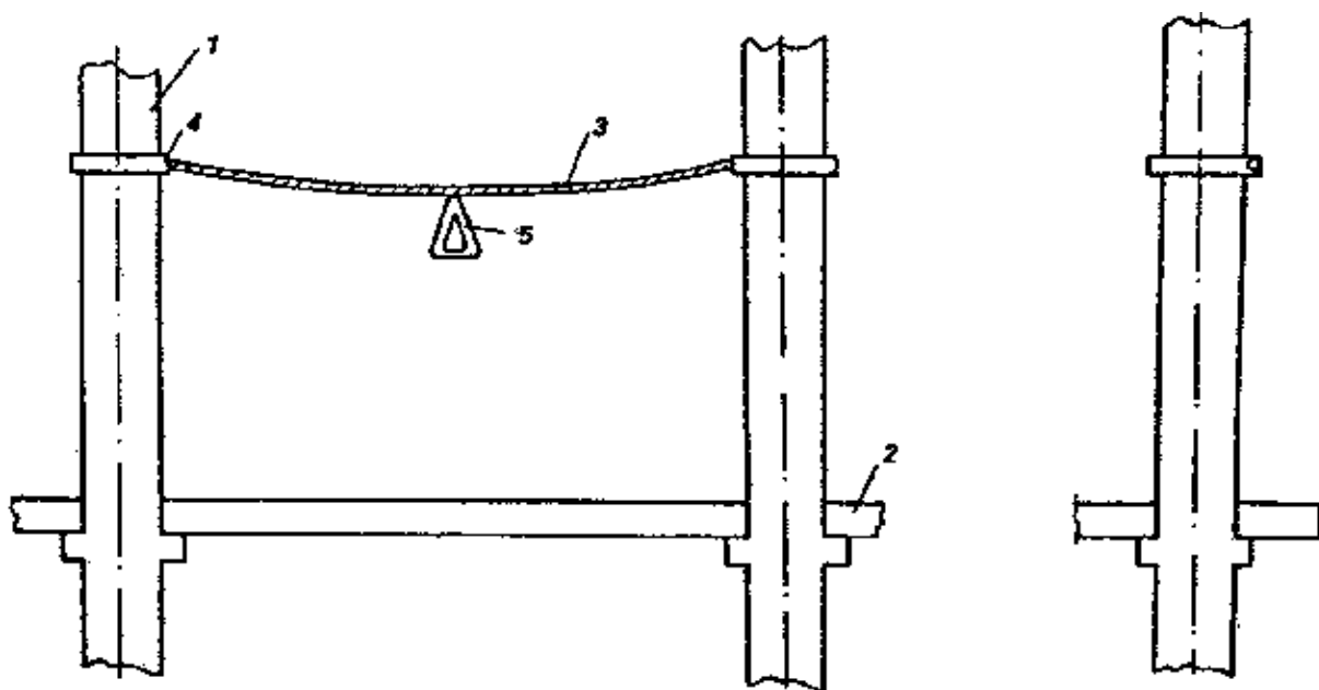
1 — колонна здания; 2 — плита перекрытия; 3 — заполнение; 4 — хомут; 5 — знак безопасности
