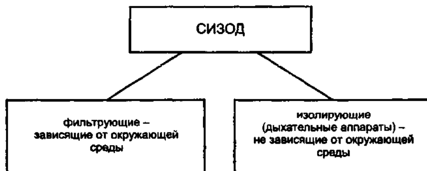
Рисунок 2 — Классификация средств индивидуальной защиты органов дыхания
