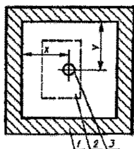
Расположение зоны удара при испытании вертикально падающим предметом
