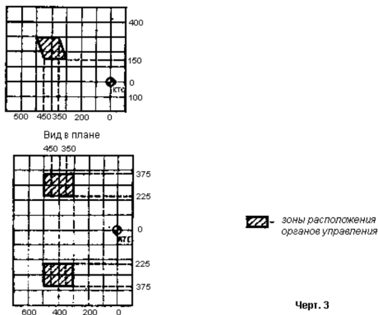
Рекомендуемые зоны расположения органов ручного управления при электрогидравлической, гидрогидравлической и других аналогичных системах управления
