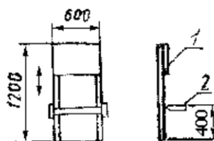
1 - стенка; 2- сиденье Черт. 3
