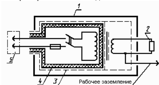
Пример выполнения изделий класса II
