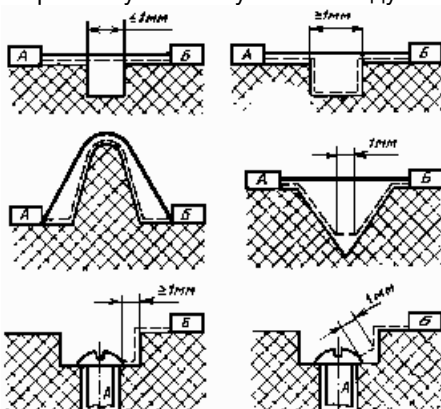
Схемы измерения путей тока утечки и воздушных зазоров
