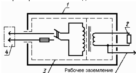
Пример выполнения изделий класса III
