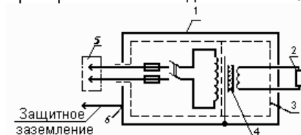
Пример выполнения изделий класса 0I
