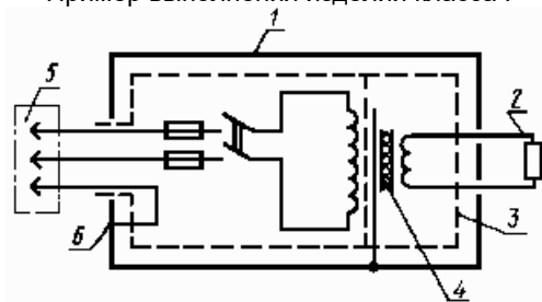
Пример выполнения изделий класса I
