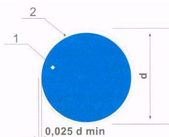
Рисунок 3 - Основа цветографического изображения и соотношение размеров предписывающих знаков пожарной безопасности
