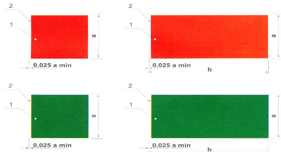
Рисунок 4 - Основа цветографического изображения и соотношение размеров указательных знаков пожарной безопасности
