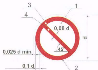
Рисунок 1 - Основа цветографического изображения и соотношение размеров запрещающих знаков пожарной безопасности
