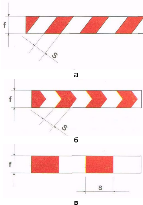
а - расположение полос наклонно; б - расположение полос зигзагообразно в виде «елочки»; в - расположение полос прямо (вертикально или горизонтально); f - поперечный размер сигнальной ленты; s - ширина полосы сигнального цвета
