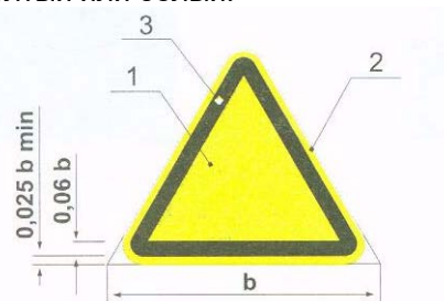
Рисунок 2 - Основа цветографического изображения и соотношение размеров предупреждающих знаков пожарной безопасности
