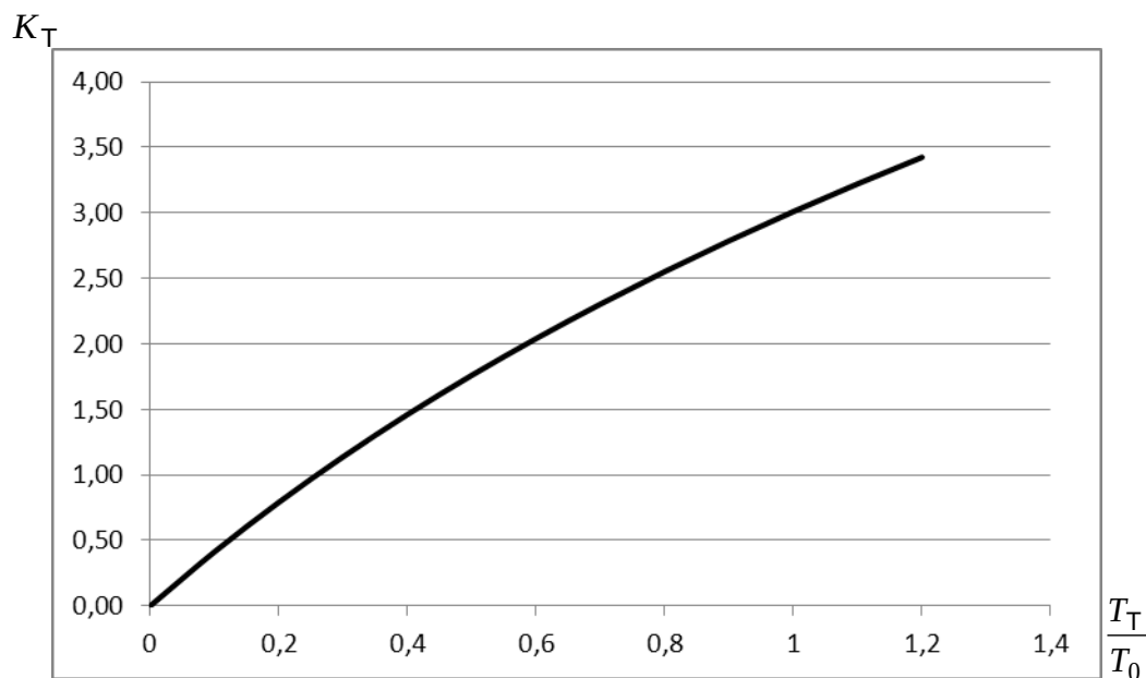
Рисунок А.1 – Зависимость K_T , дБ, от T_T/T_0
