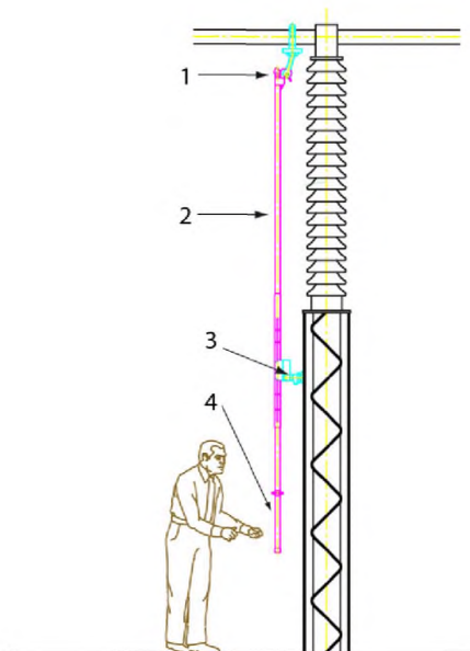
1 — копьевой контакт на проводнике; 2 — копье; 3 — неподвижная точка заземления; 4 — изолированная ручка
