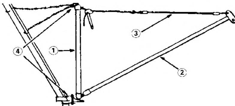
1 — мачта; 2 — стрела; 3 — штанга подвешной тяги; 4 — точки крепления (к электрической опоре)
