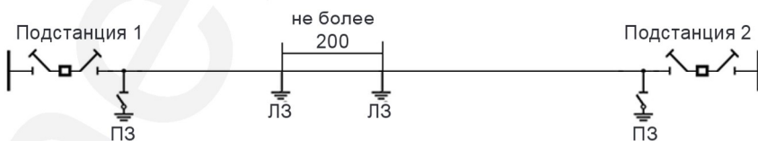
Рисунок К.5 – ВЛ 0,4–10,0 кВ разземлена в РУ и заземлена на линейные заземления, установленные с обеих сторон от места работы
