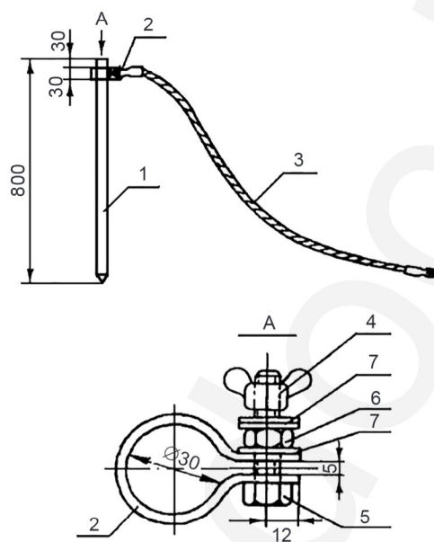
Рисунок М.4 – Стержневой заземлитель
