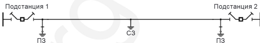
Рисунок К.4 – ВЛ заземлена в РУ и в одном или нескольких местах ВЛ на специальное заземление
