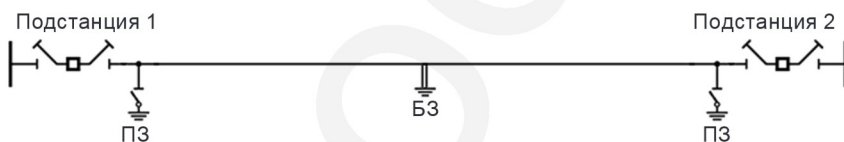
Рисунок К.3 – ВЛ разземлена во всех РУ и заземлена на базовое заземление
