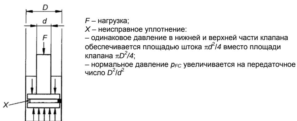
Рисунок 13 – Давление в цилиндре; разгерметизация
