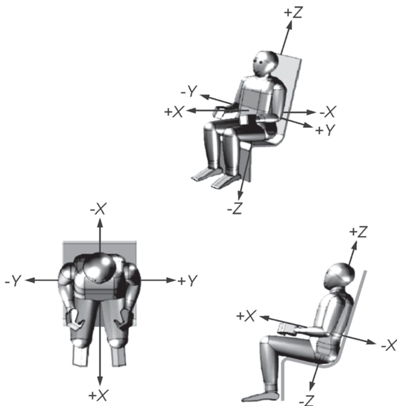
Рисунок А.1 — Система координат тела человека
