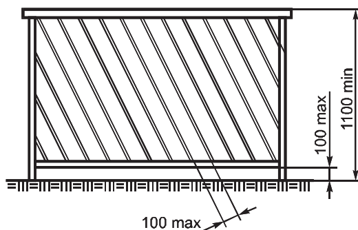
а) Ограждение с наклонным расположением внутренних элементов
