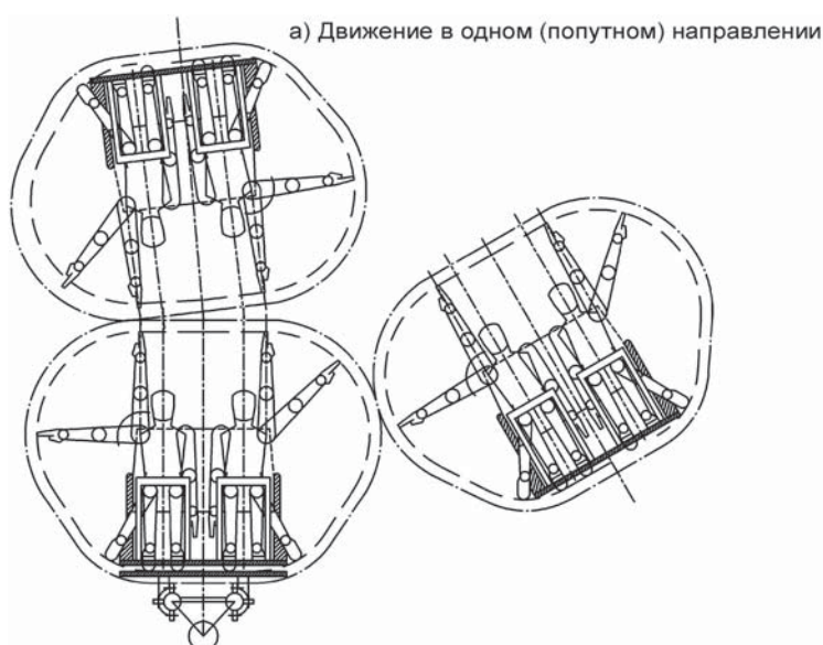
Рисунок 8, лист 1 — Контур безопасности для движущихся пассажирских модулей
