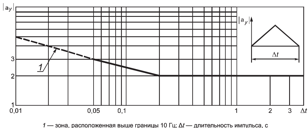
Рисунок Б.1 — Допустимое ускорение сиденья |a_y| в зависимости от длительности импульса
