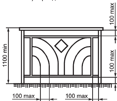
в) Ограждение с декоративными элементами
