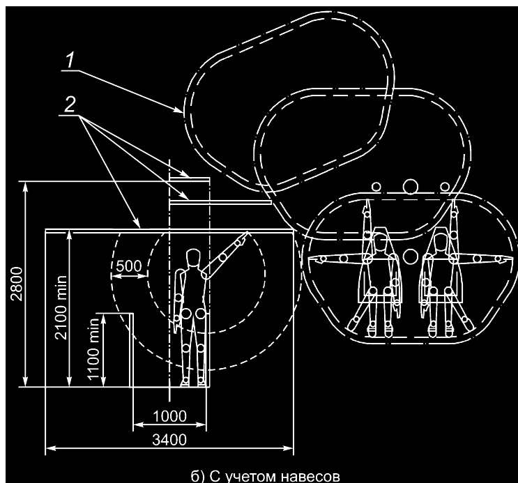
1 — контур безопасности пассажирского модуля; 2 — навес
