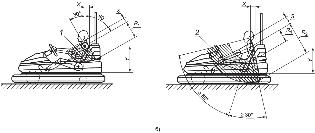
Рисунок 15 — Сталкивающиеся электромобили
