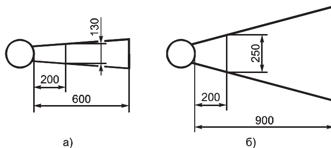
Рисунок 2 — Размеры спиральных и винтовых лестниц
