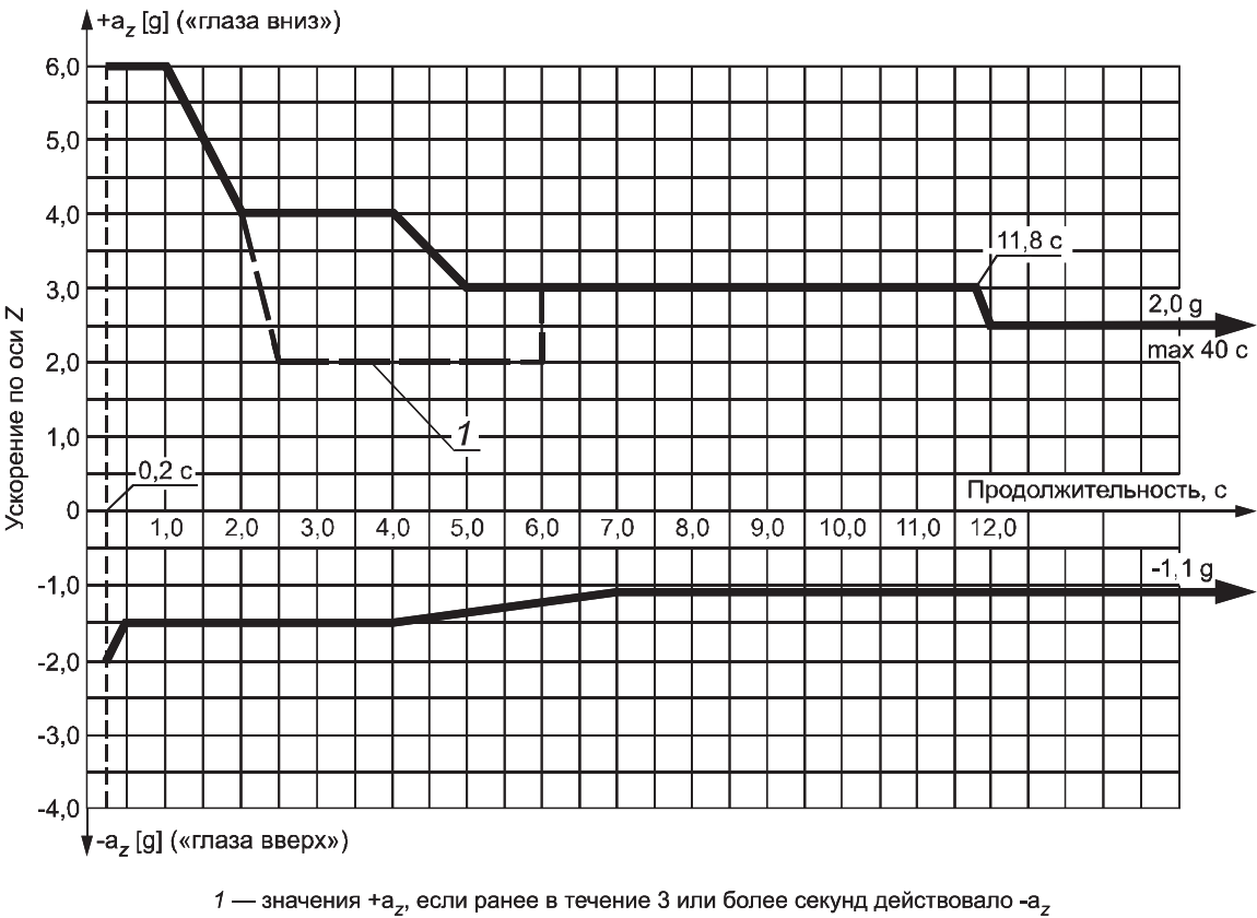
Рисунок А.4 — Пределы по времени для ускорений в направлении Z (параллельно позвоночнику)
