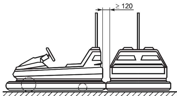
Рисунок 9 — Минимальный зазор для свободно перемещающихся пассажирских модулей
