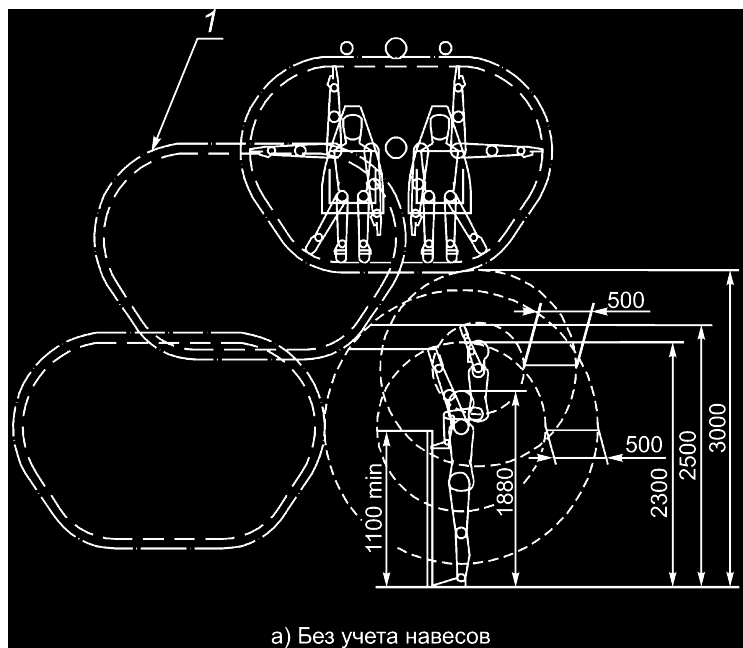
1 — контур безопасности пассажирского модуля
