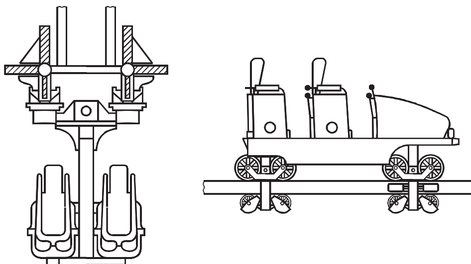
а) Атракцион с направляющими
