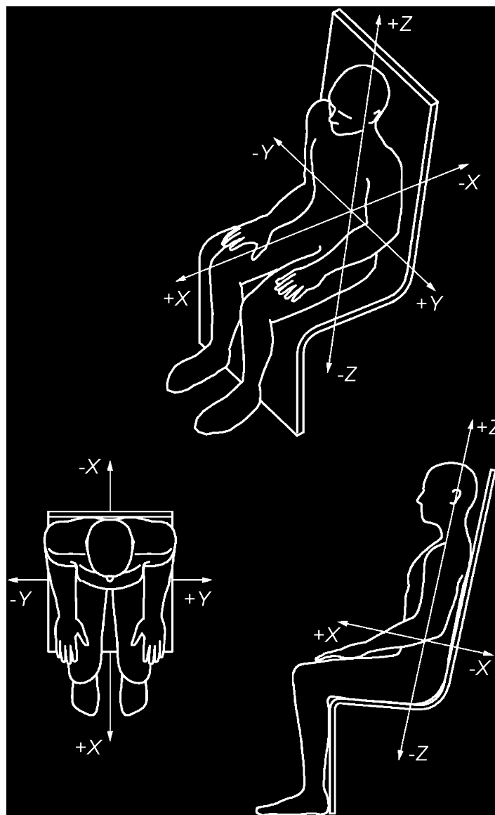
Рисунок 10 — Система координат для ускорений
