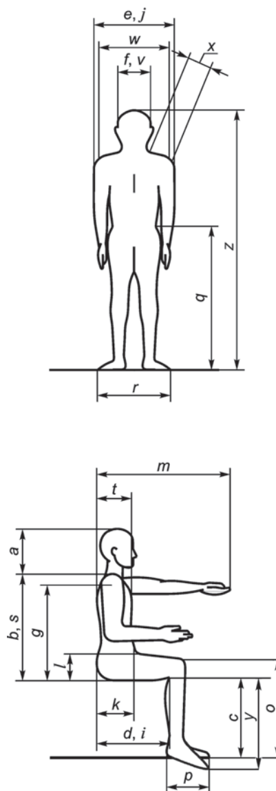
Рисунок Д.1 — Размеры тела (таблица Д.2)
