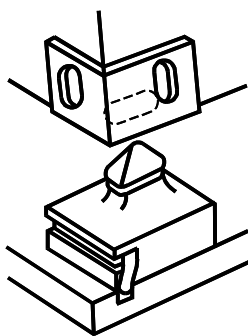
Рисунок 7 – Поворотный штыковой замок
