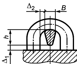
Рисунок 1 — Зацепка грузов крюками за строповочные элементы
