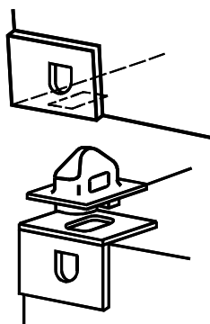
Рисунок 10 – Штыковой упор
