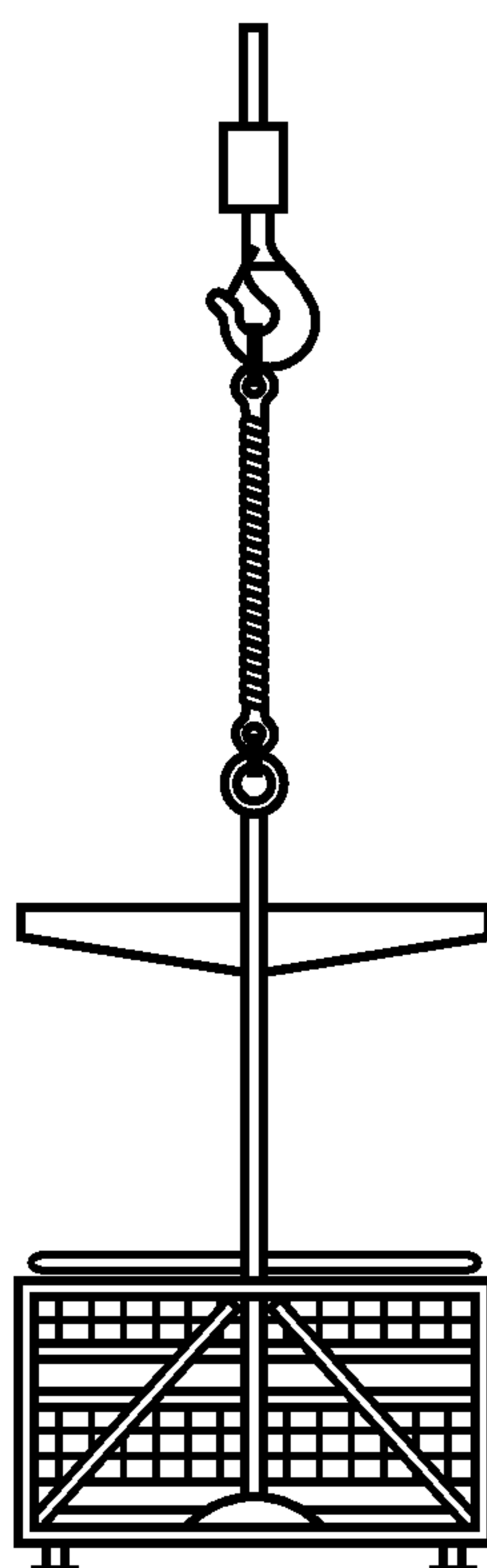
Рисунок 3 — Кабина (люлька) с одним стропом
