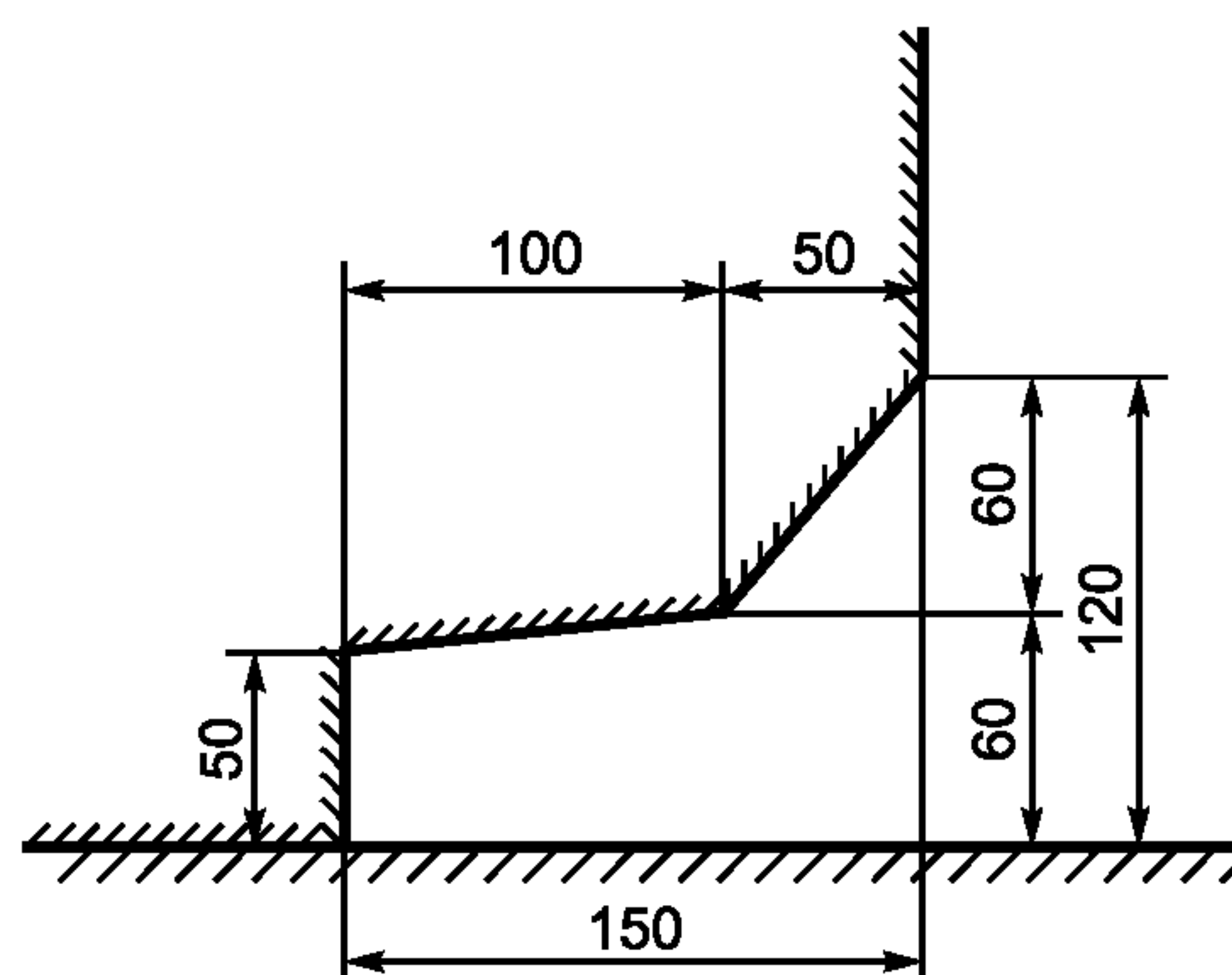
Рисунок 4 — Минимальные размеры пространства для ног
