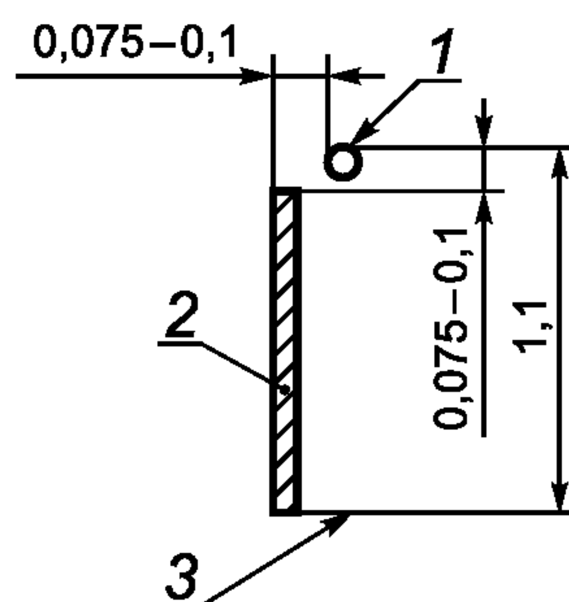
1 — поручень; 2 — боковое ограждение; 3 — пол (настил) кабины (люльки)
