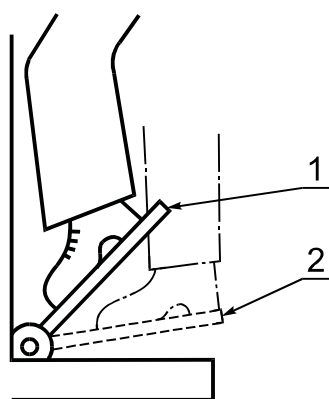
1 — тормоз зажат; 2 — тормоз отпущен
